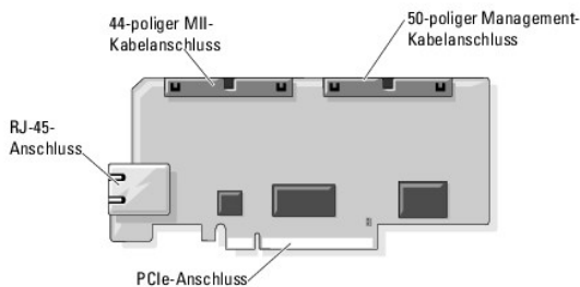
Abbildung 1-1. DRAC 5-Hardwarefunktionen
